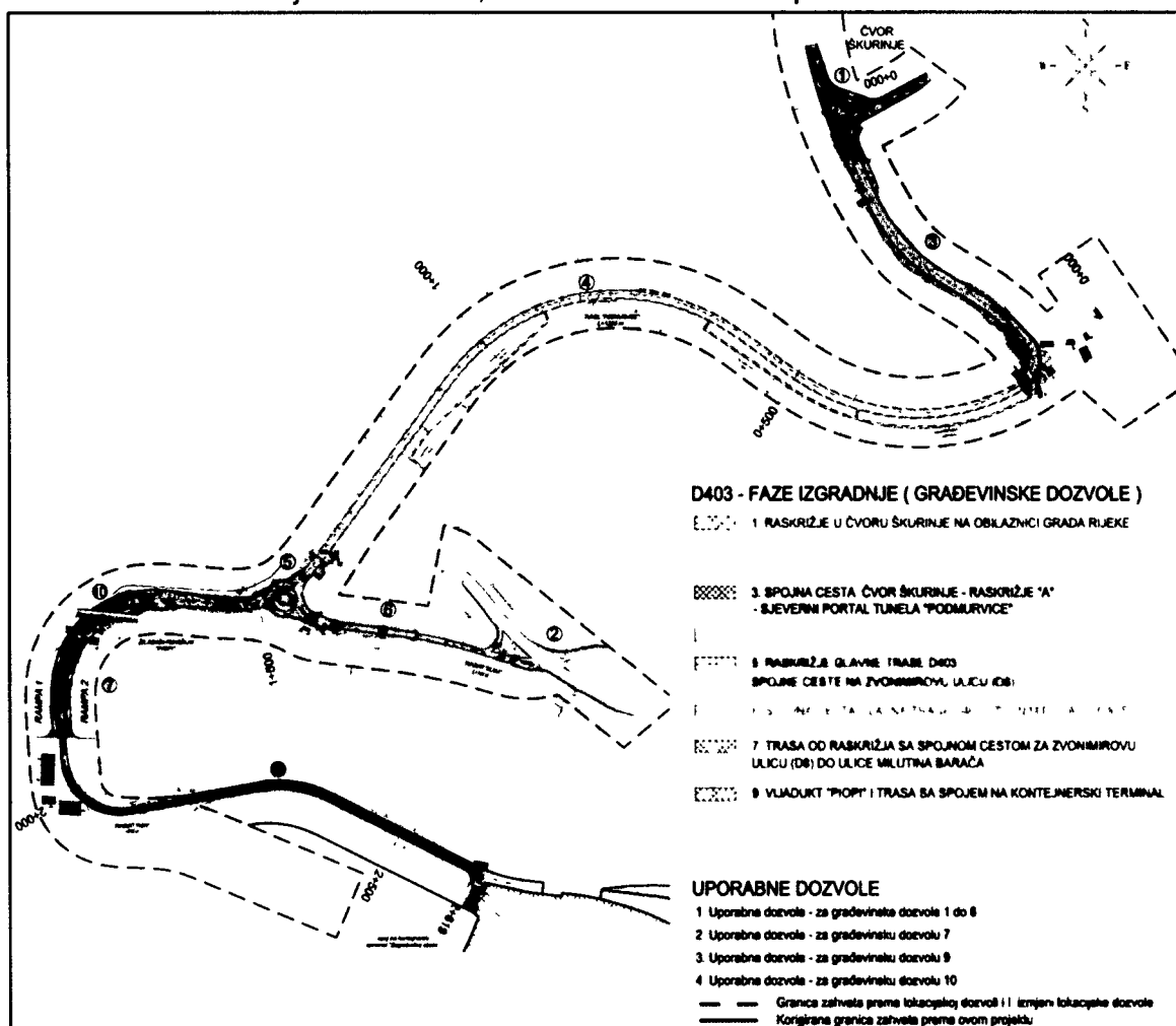
Podjela ceste D403 na faze
