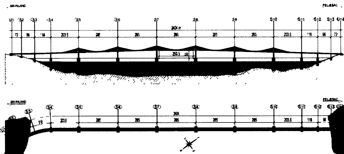
Osnovna skica mosta
