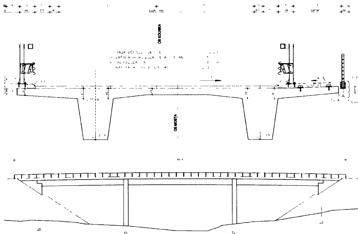
Poprečni presjek i pogled na most Odra na spojnoj cesti čvor Sisak (A1) – Sisak
